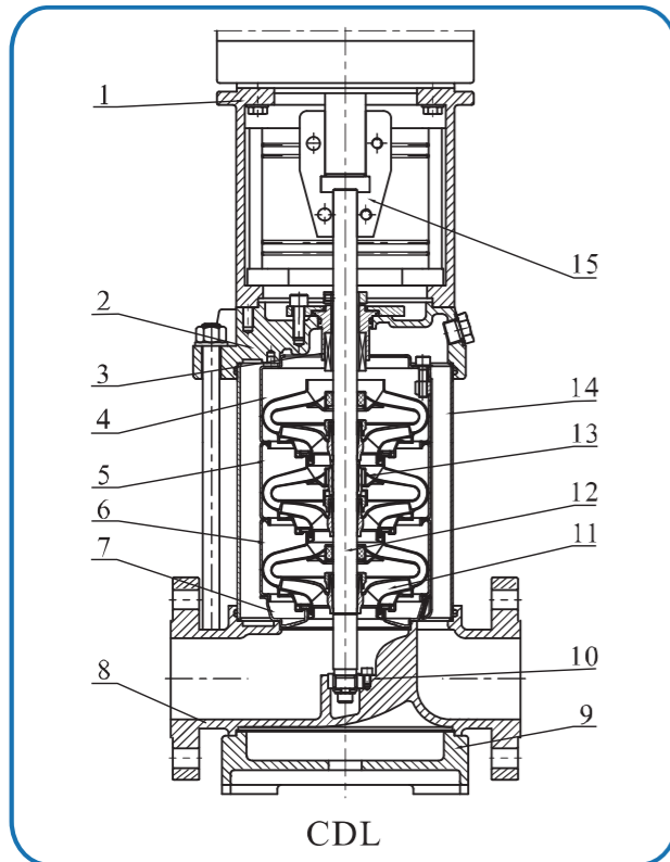
截面图 CDL,CDLF32,42,65,85
