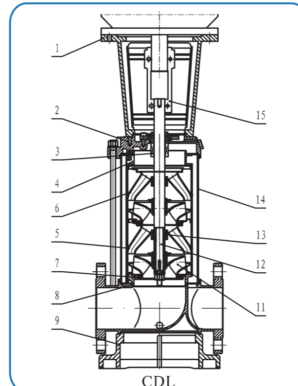
截面图 CDL,CDLF120,150,200
