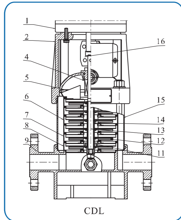
截面图 CDL,CDLF1,2,3,4
