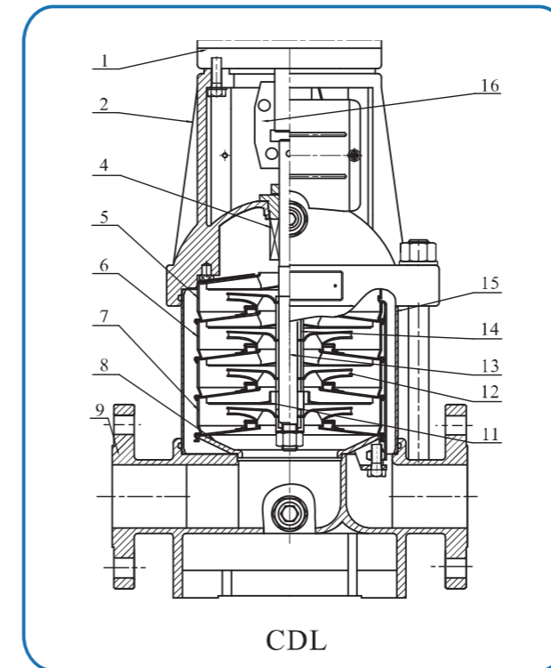
截面图 CDL,CDLF8,10,12,15,20
