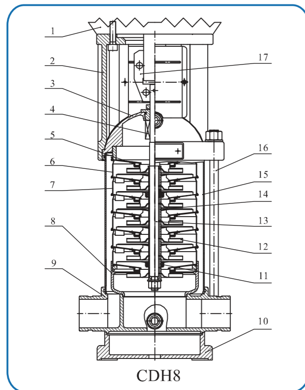
截面图 CDH8,12,15,20
